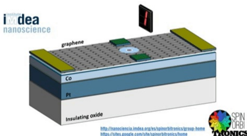
Principio de funcionamiento de la memoria basada en grafeno y skyrmions pasando. / IMDEA Nanociencia
