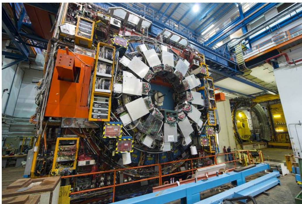
Detector CDF de Tevatron. / Fermilab
